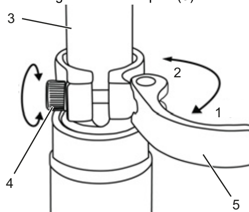
Afbeelding 102: Snelspanner van de zadelpen openen
