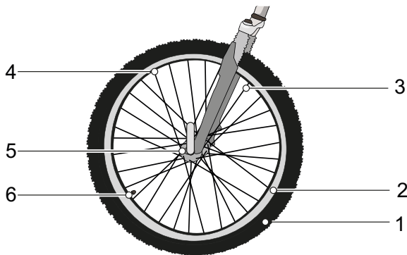
Afbeelding 16: Zichtbare componenten van het wiel
