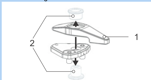
Afbeelding 82: Vergrendelhendel met grondplaat verbinden
