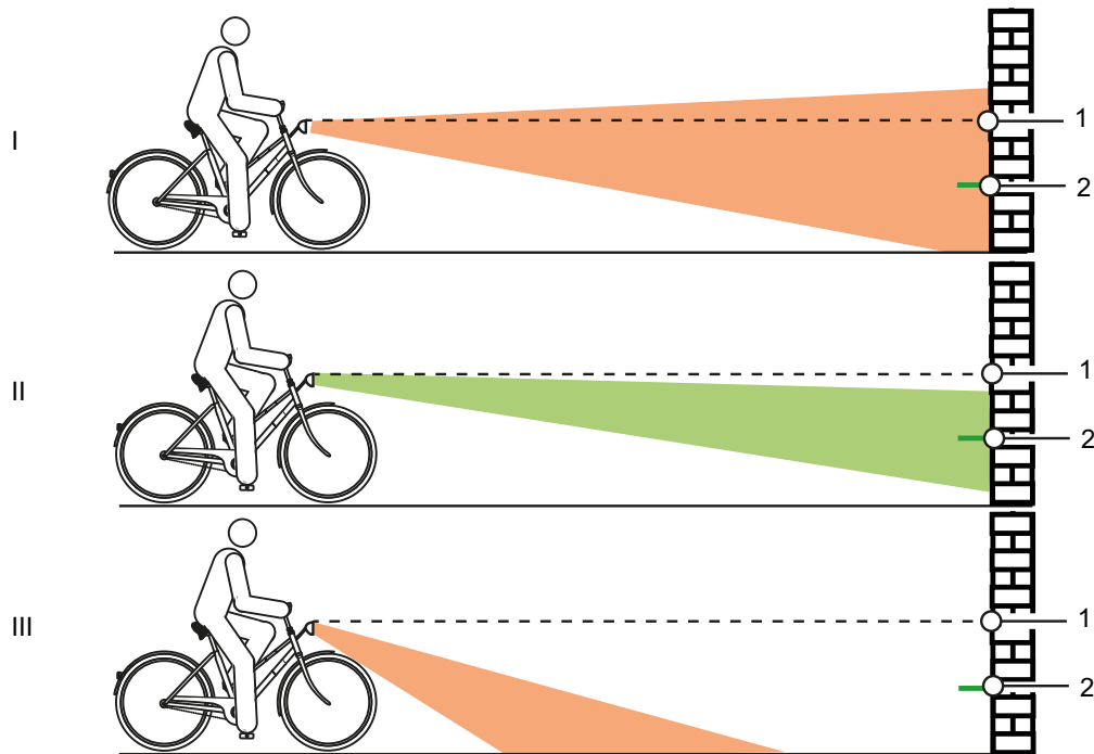
Afbeelding 187: Te hoog (1), correct (2) en te laag (3) afgestelde verlichting
