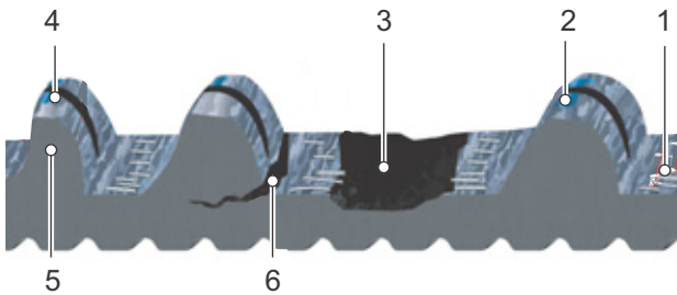
Afbeelding 176: Tekenen van slijtage op een riem
