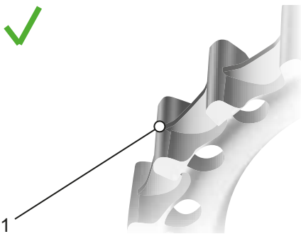
Afbeelding 177: Optimaal tandprofiel
