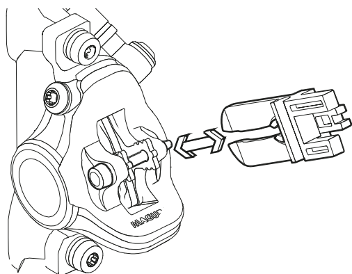
Afbeelding 62: Transportbeveiliging bevestigen
