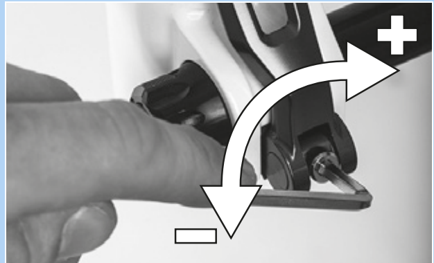
Afbeelding 194: Spankracht van de snelspanner afstellen
