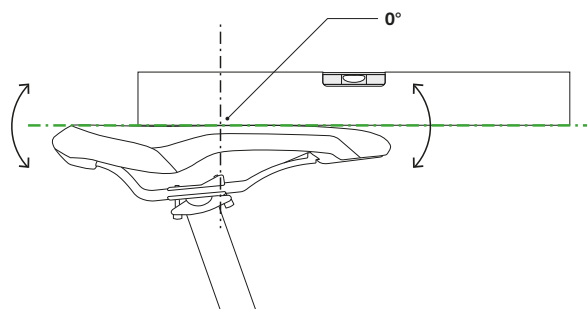
Afbeelding 106: Horizontale zadelhoek met 0° neiging in het midden van het zadel
