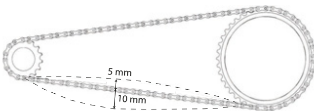
Afbeelding 166: Voorbeeld kettingspanning controleren: 5 mm omhoog, 10 mm omlaag = 15 mm uitwijking
