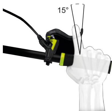
Afbeelding 118: Stand remhendel
