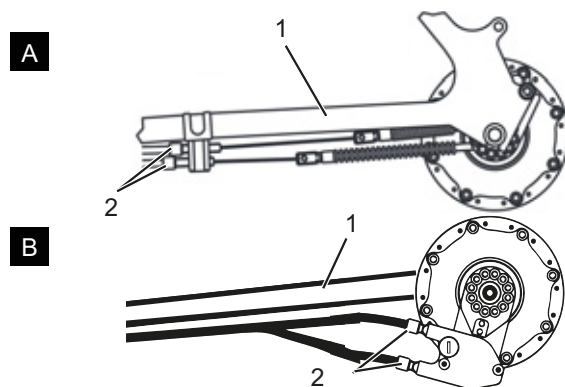
Afbeelding 191: Afstelwartels (2) van twee alternatieve uitvoeringen (A en B) van een versnelling met dubbele bowdenkabelbediening aan de achterbrug (1)
