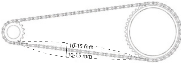
Afbeelding 188: Kettingspanning controleren
