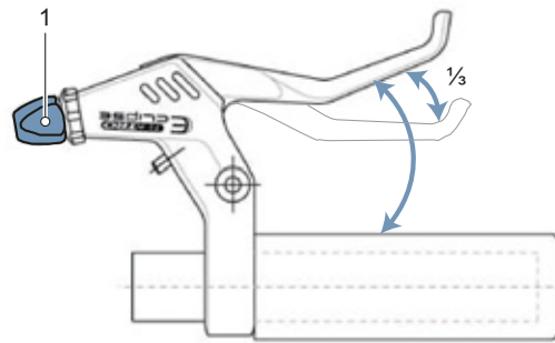
Afbeelding 165: Stelschroef (1) draaien tot het remmen na \frac{1}{3} van de afgelegde weg van de handrem inzet
