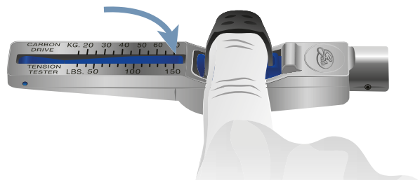
Afbeelding 180: Wijsvinger op instrument
