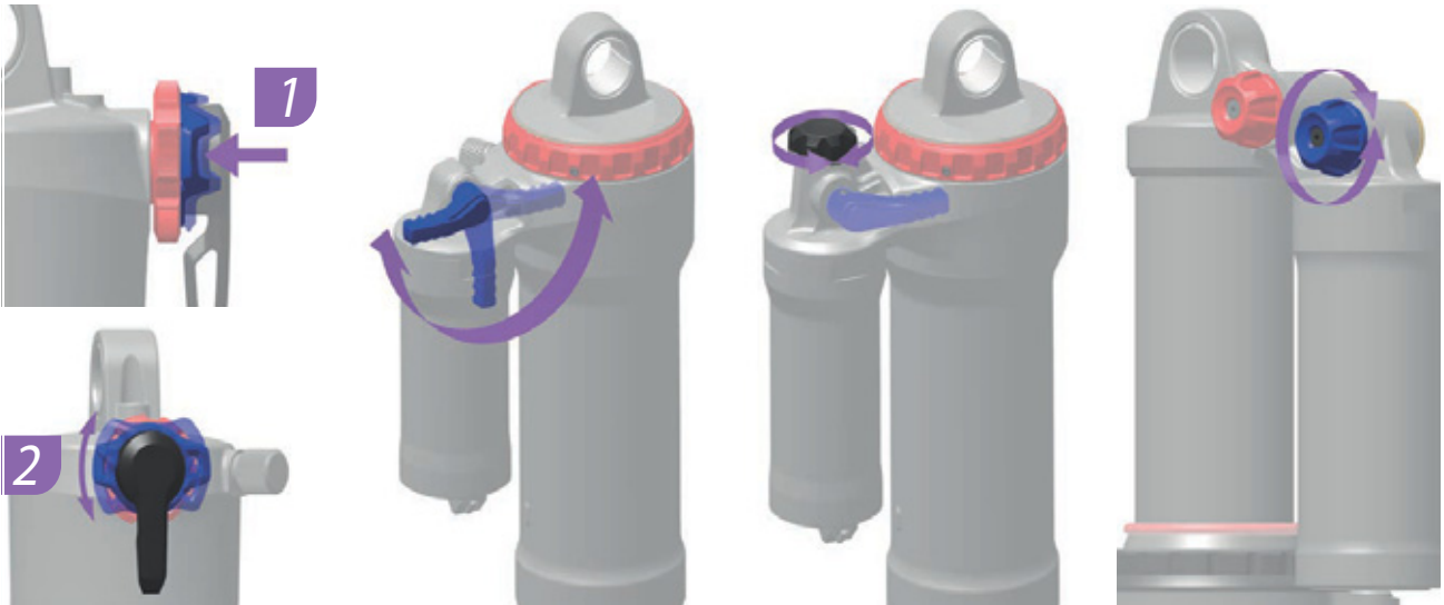
Afbeelding 226: Locatie en vorm van de drukdemperafsteller (blauw) is afhankelijk van het model
